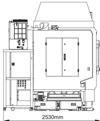
左视图
